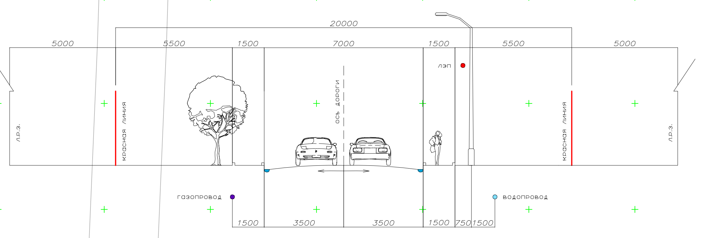
Схема поперечного профиля улицы А-А. М 1:100
